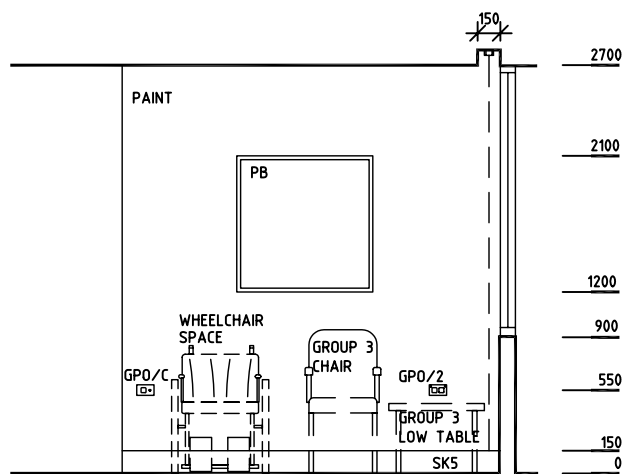
ELEVATION 3
