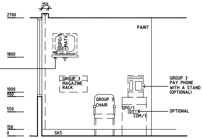
ELEVATION 2
