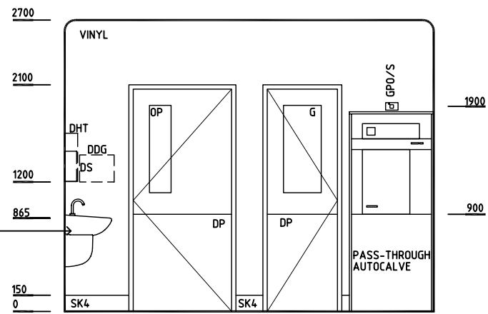
ELEVATION 2
