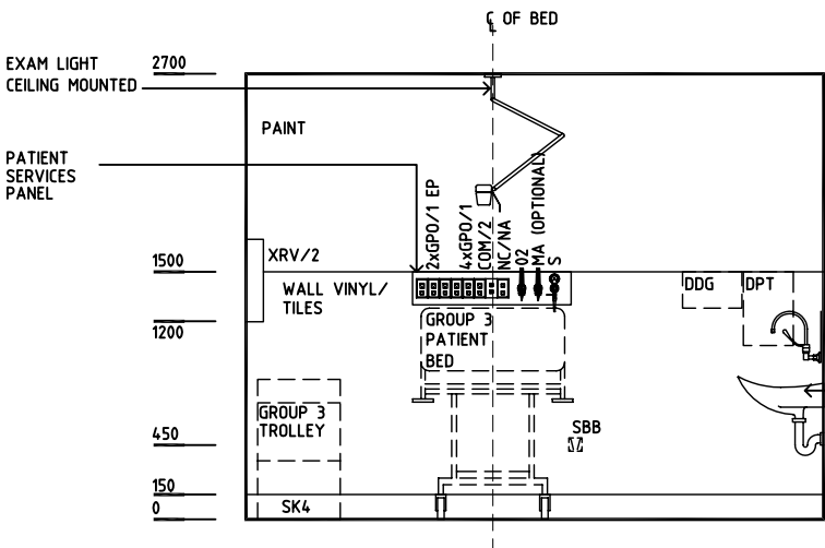
ELEVATION 1
