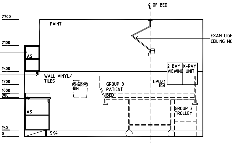
ELEVATION 4
