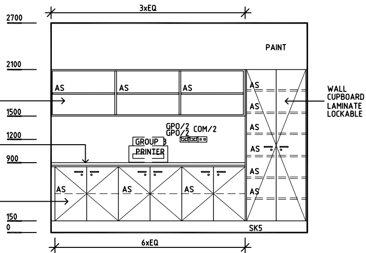
ELEVATION 4
