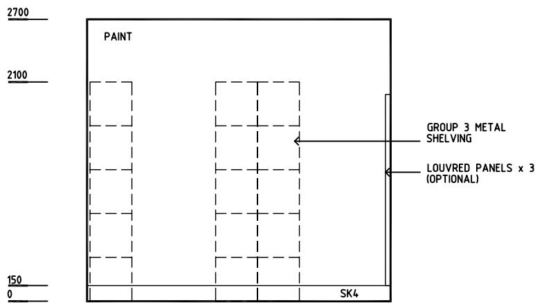
ELEVATION 1
