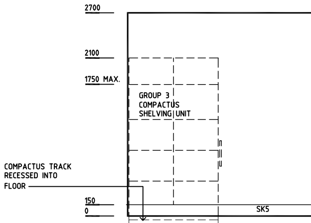
ELEVATION 2
