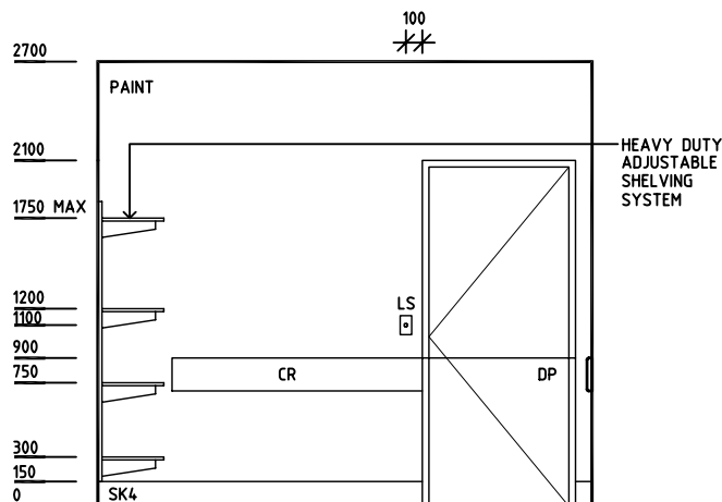
ELEVATION 3
