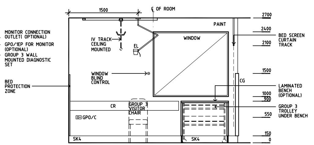
ELEVATION 2
