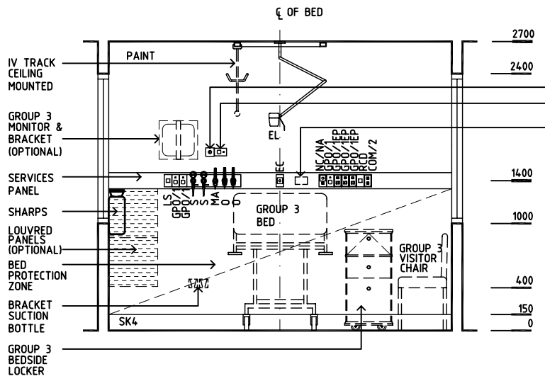
ELEVATION 1
