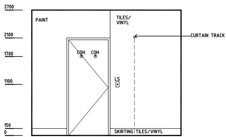
ELEVATION 2
