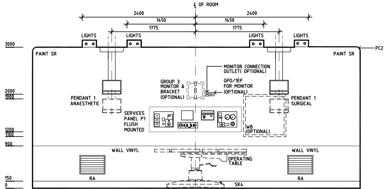
ELEVATION 2
