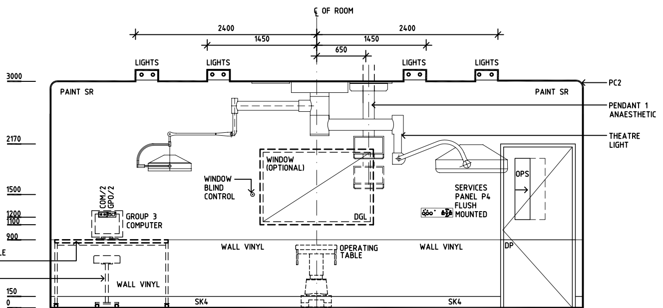
ELEVATION 1
