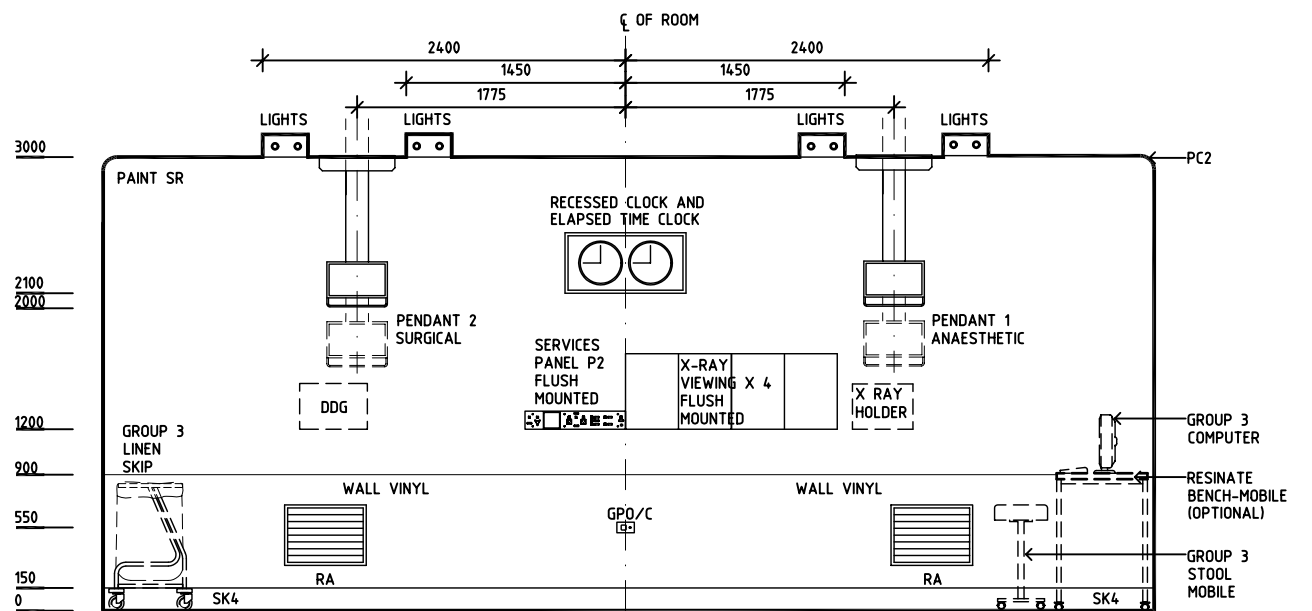
ELEVATION 4
