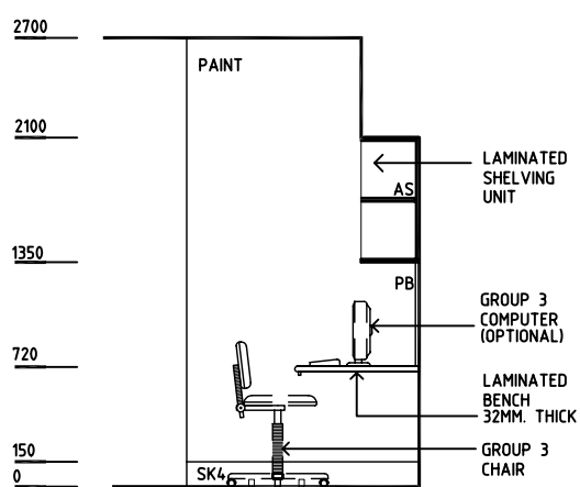
ELEVATION 1
