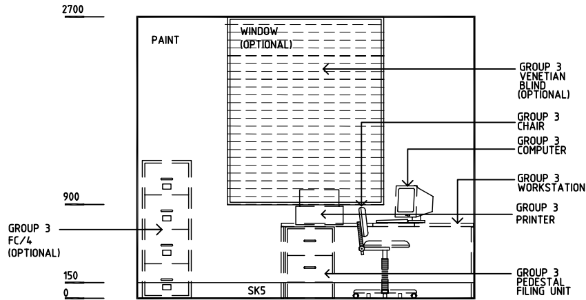
ELEVATION 1
