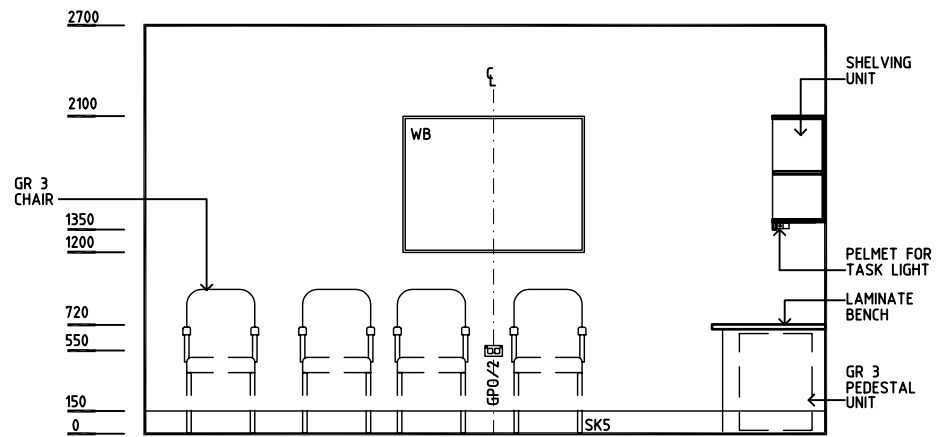
ELEVATION 4
