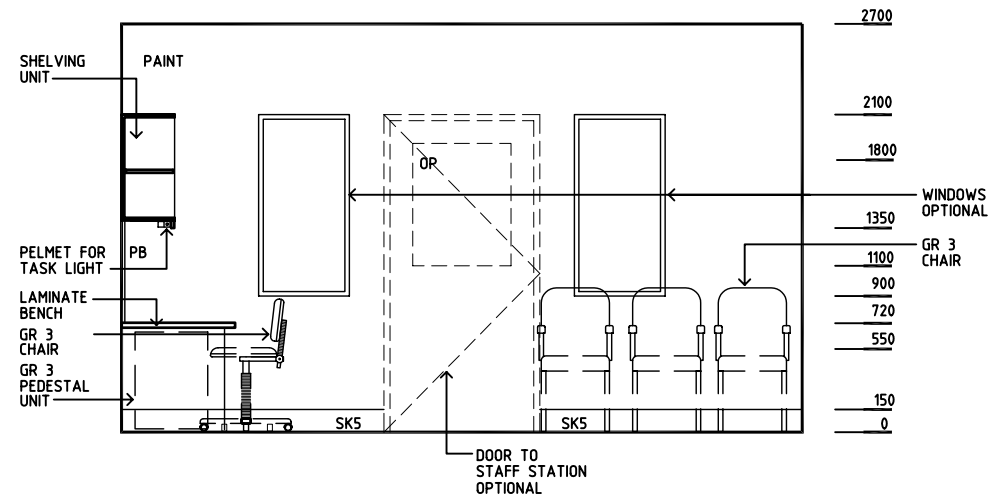
ELEVATION 2
