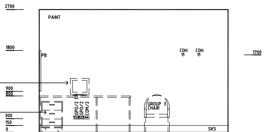
ELEVATION 2
