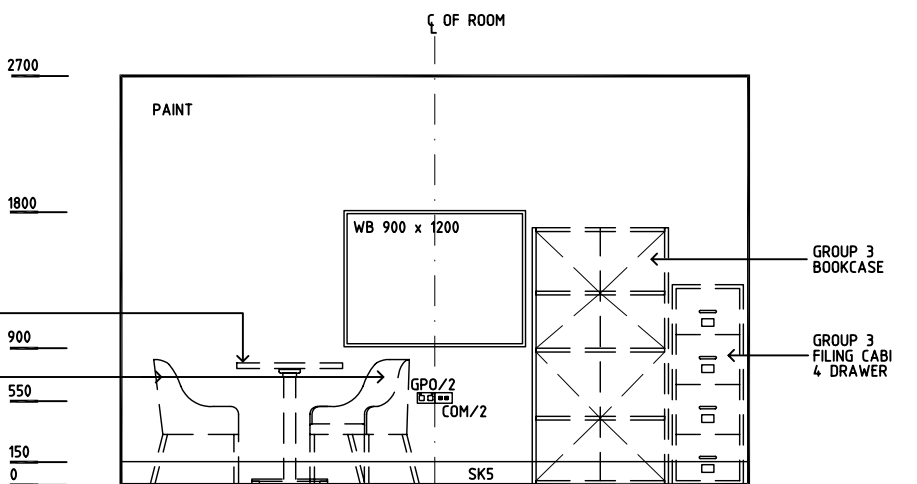
ELEVATION 4
