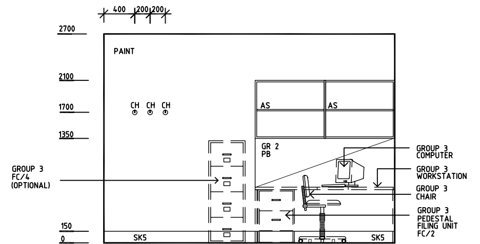
ELEVATION 4
