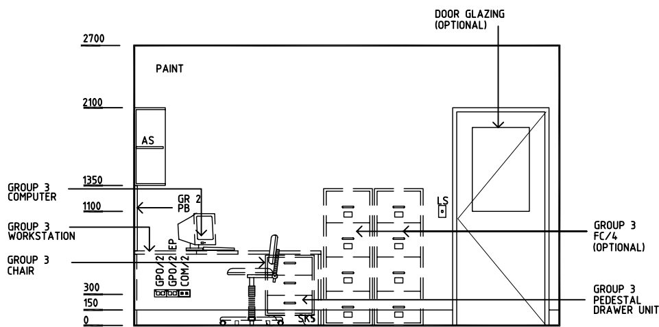
ELEVATION 3
