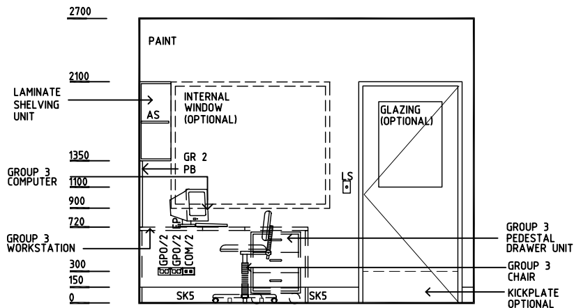
ELEVATION 3
