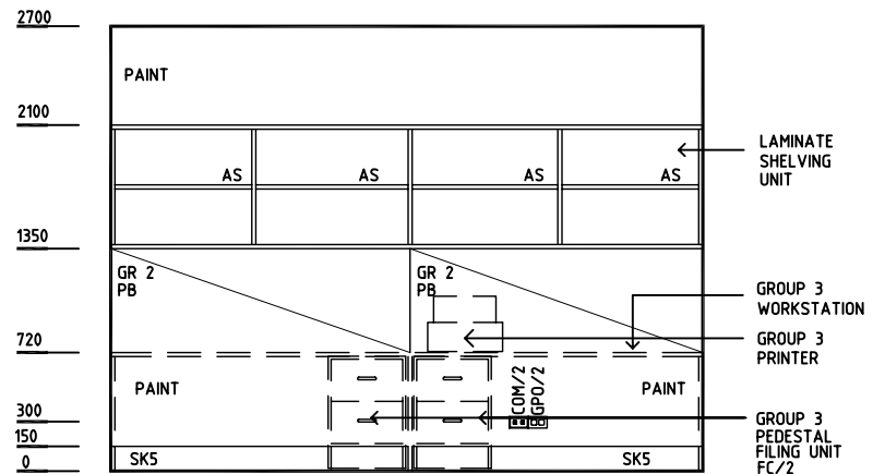
ELEVATION 2
