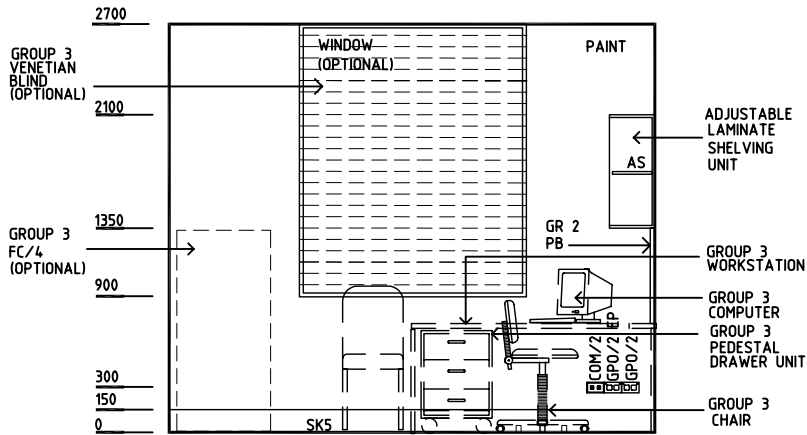
ELEVATION 1
