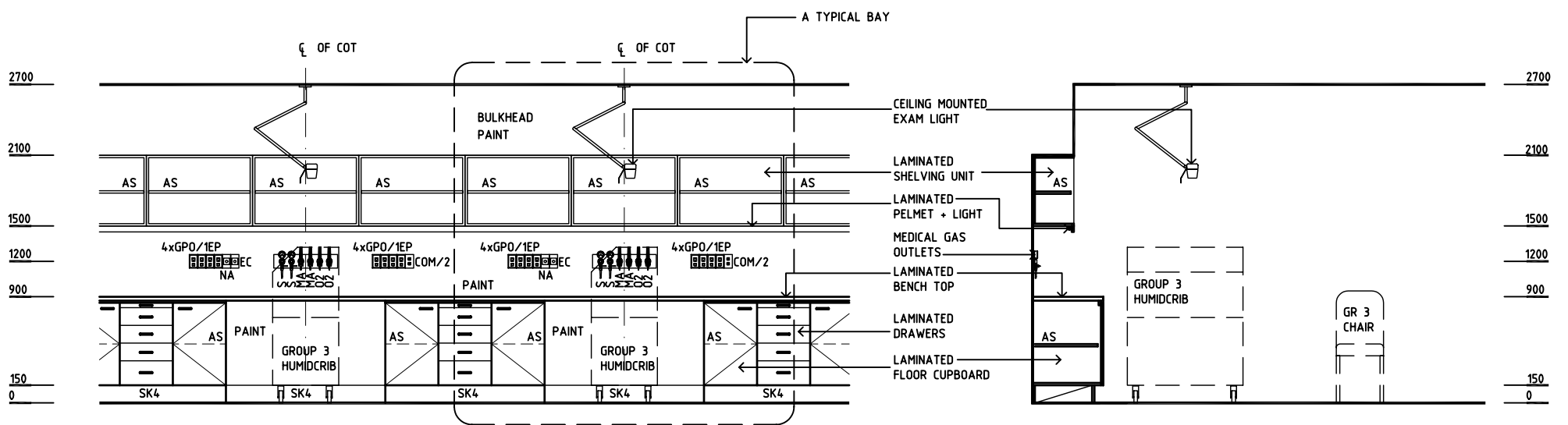
ELEVATION 1
