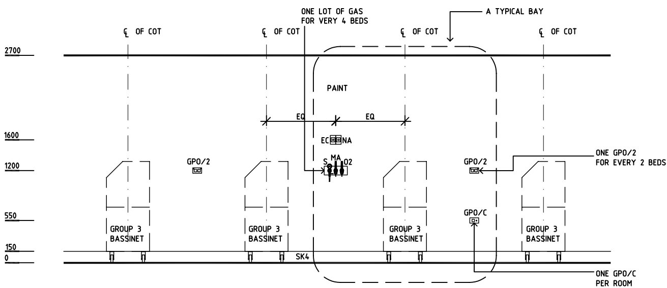
ELEVATION 1
