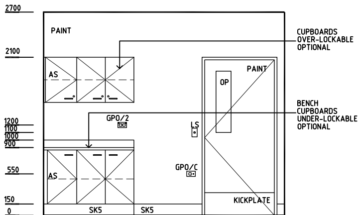
ELEVATION 3
