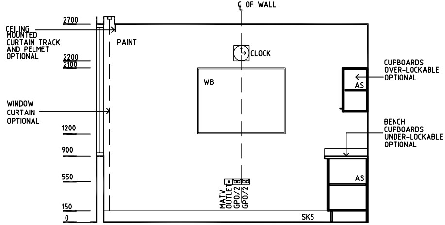
ELEVATION 2
