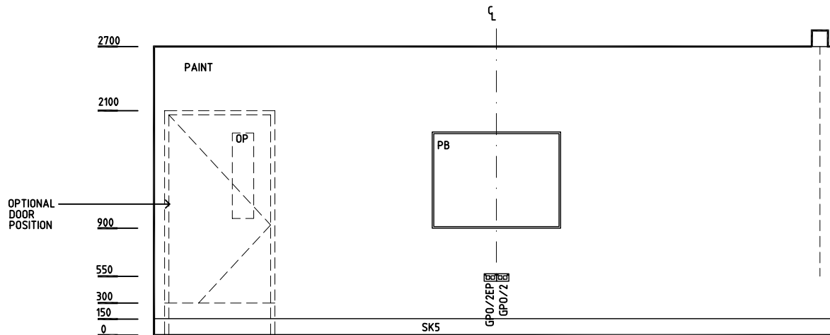
ELEVATION 4
