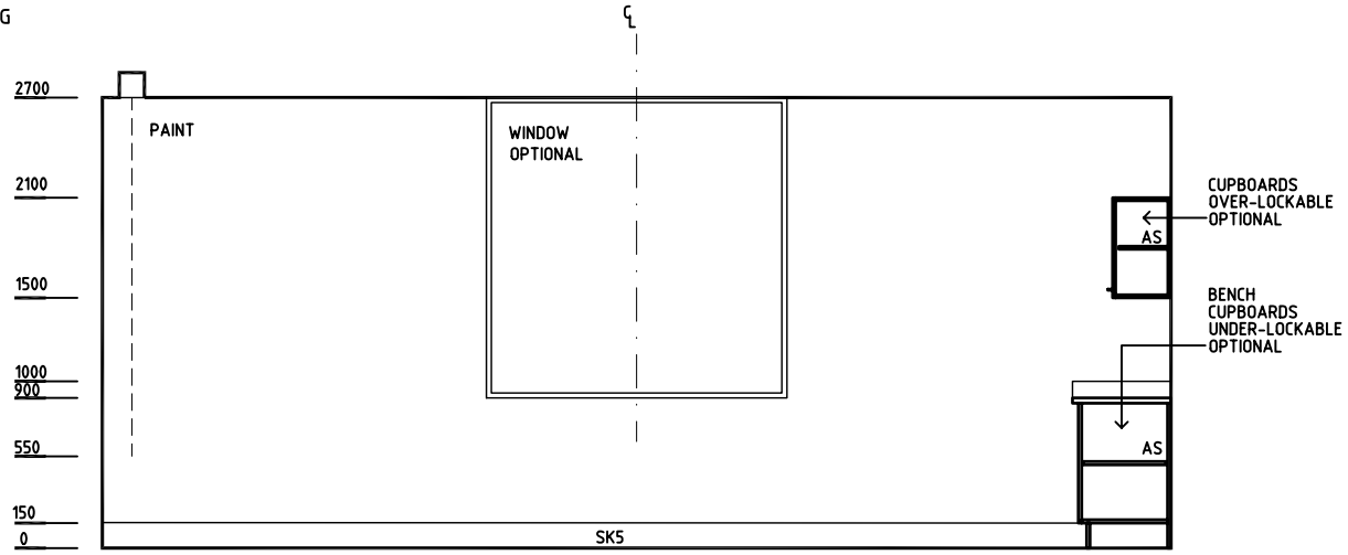
ELEVATION 2
