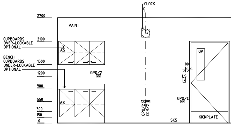
ELEVATION 3
