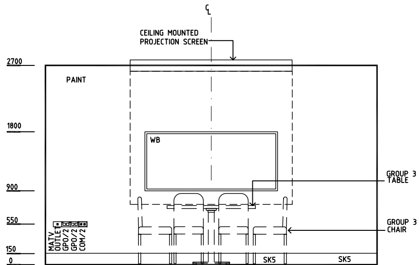
ELEVATION 1
