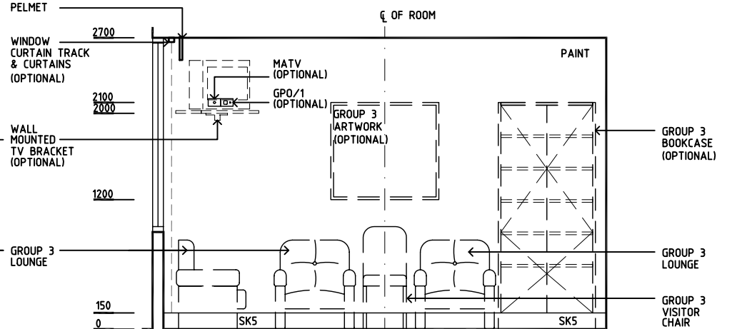
ELEVATION 2
