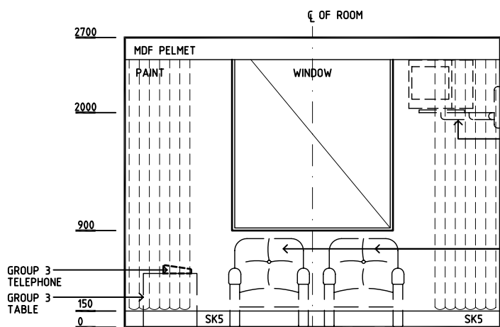
ELEVATION 1
