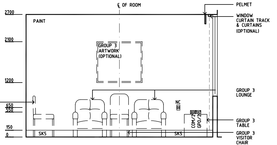
ELEVATION 4
