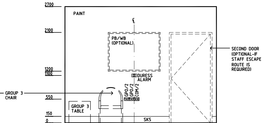
ELEVATION 4
