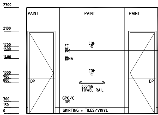
ELEVATION 1
