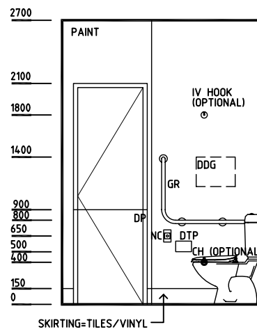
ELEVATION 2
