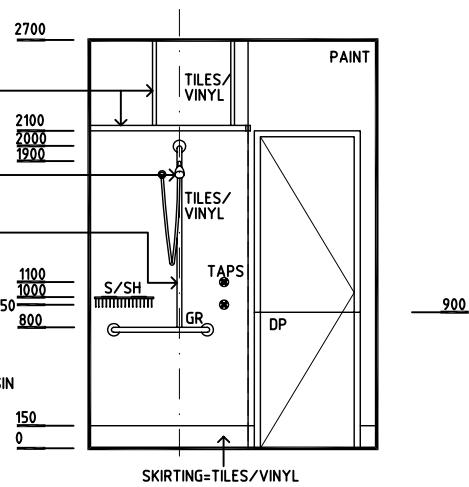
ELEVATION 4
