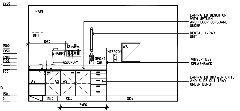
ELEVATION 2
