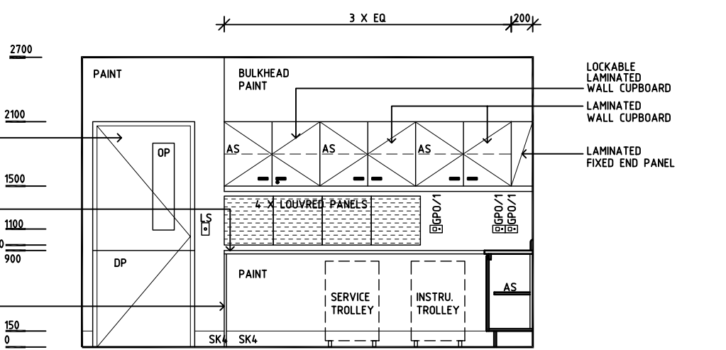
ELEVATION 4
