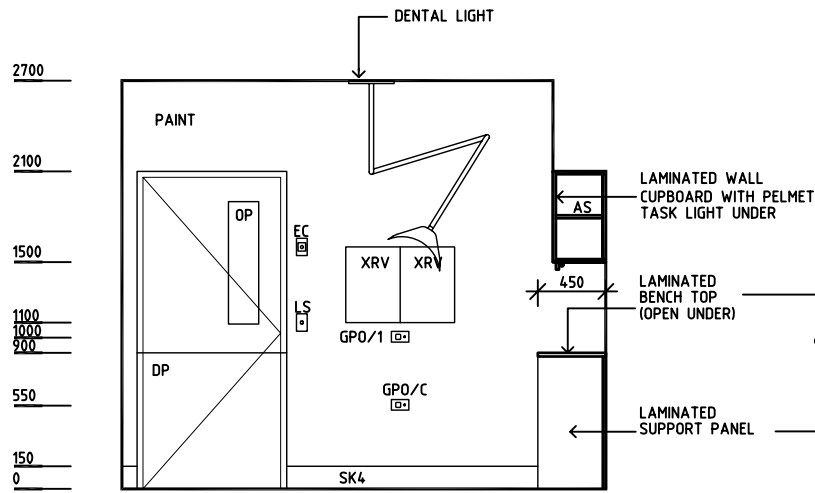
ELEVATION 3
