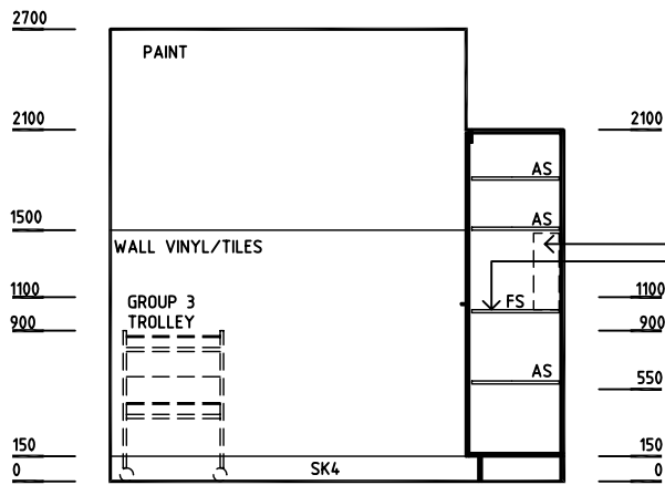
ELEVATION 1
