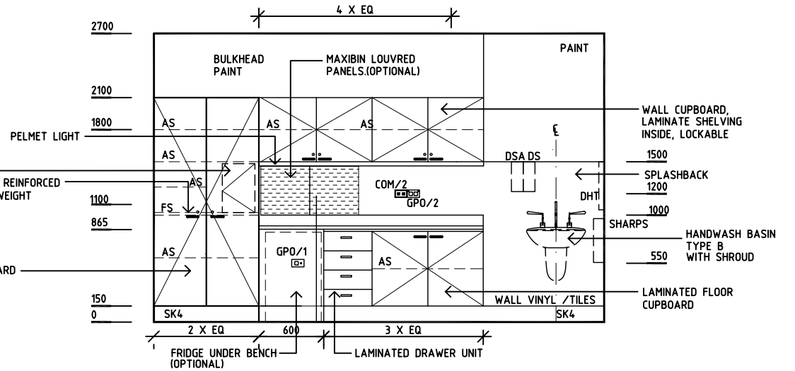
ELEVATION 2
