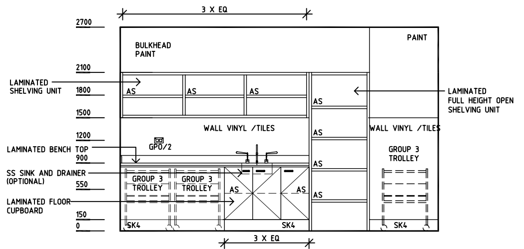
ELEVATION 4
