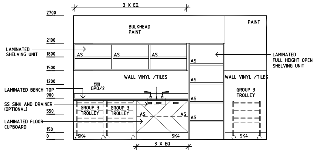
ELEVATION 2
