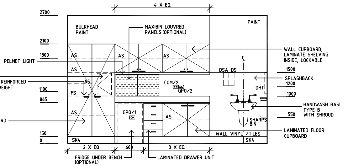
ELEVATION 2
