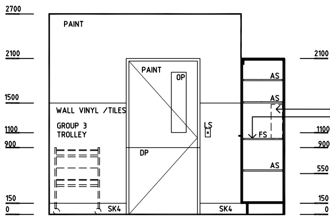
ELEVATION 1
