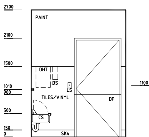
ELEVATION 3
