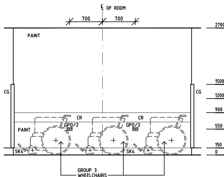
ELEVATION 2
