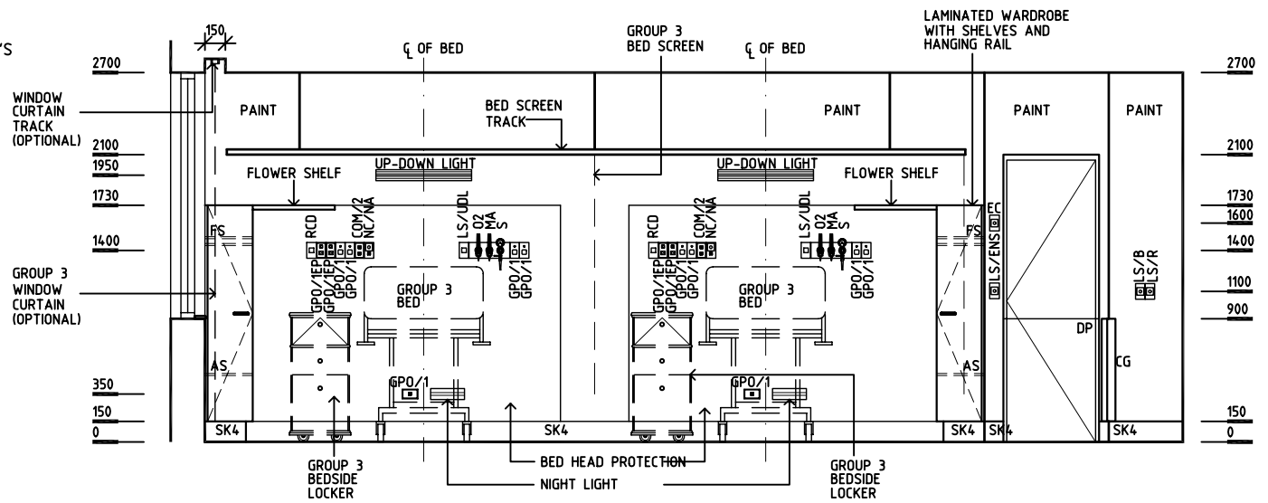
ELEVATION 2
