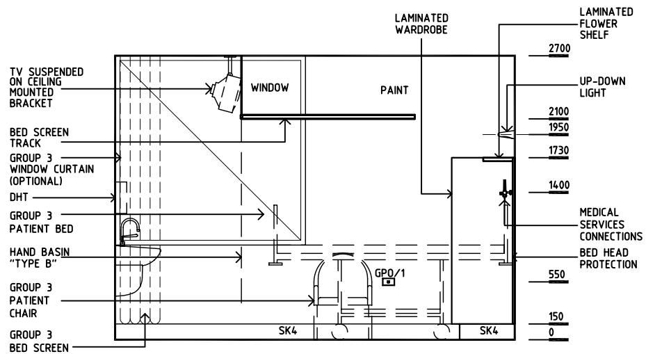
ELEVATION 1
