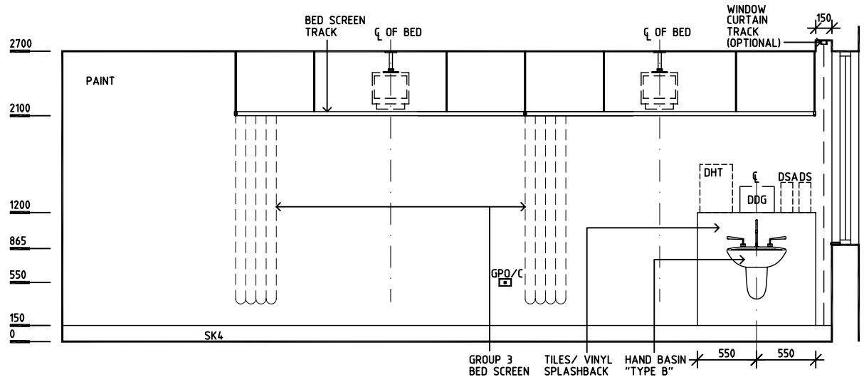
ELEVATION 4
