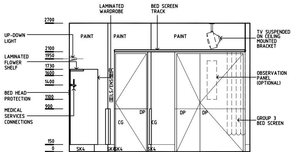
ELEVATION 3
