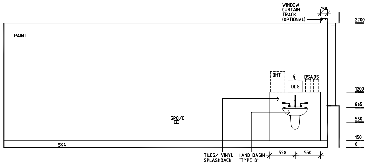
ELEVATION 4
