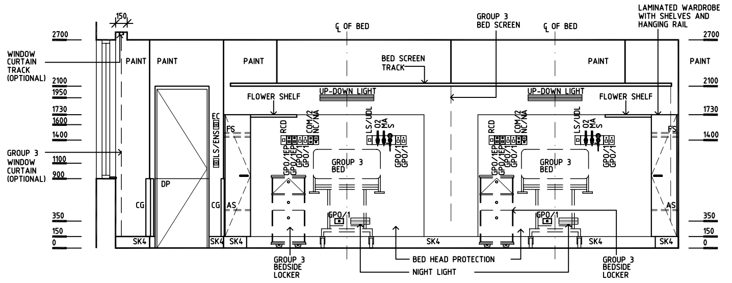
ELEVATION 2
