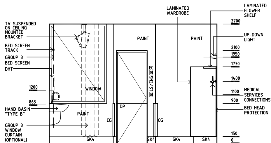
ELEVATION 1
