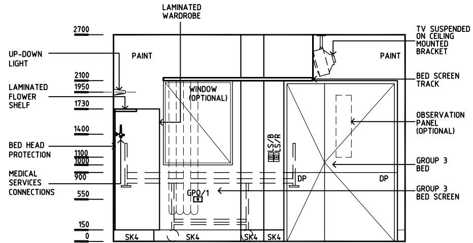
ELEVATION 3
