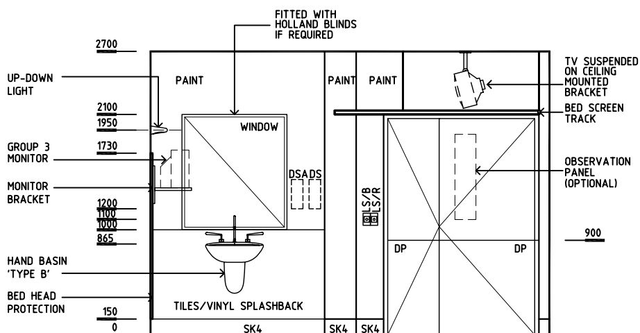
ELEVATION 1
