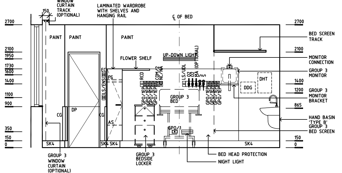
ELEVATION 2
