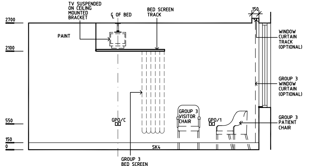
ELEVATION 4
