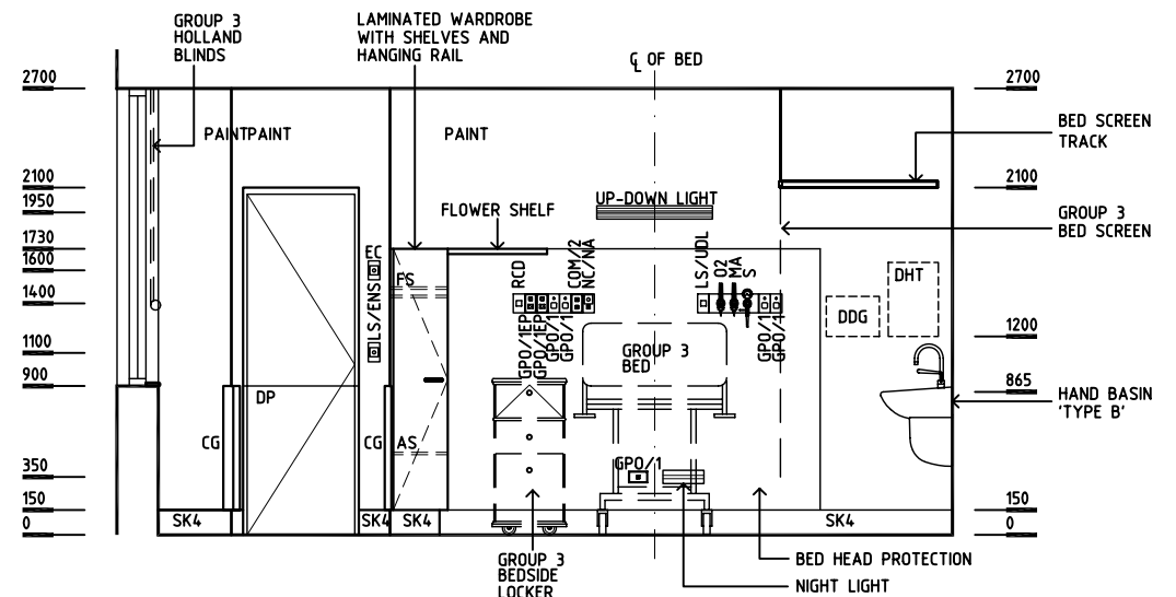
ELEVATION 2
