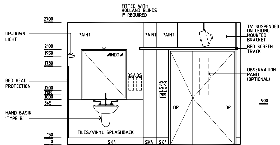
ELEVATION 3
