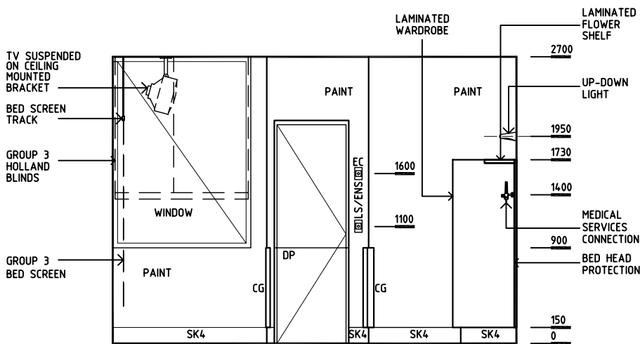
ELEVATION 1
