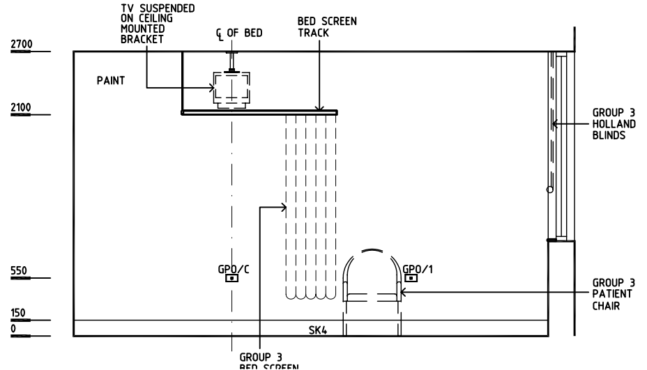
ELEVATION 4
