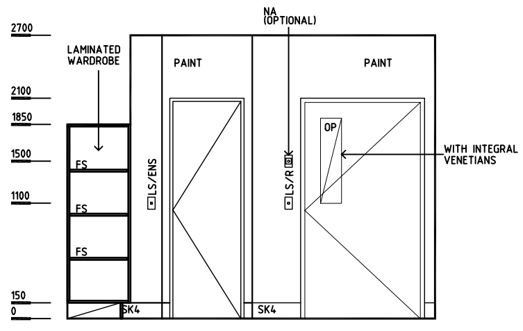
ELEVATION 3
