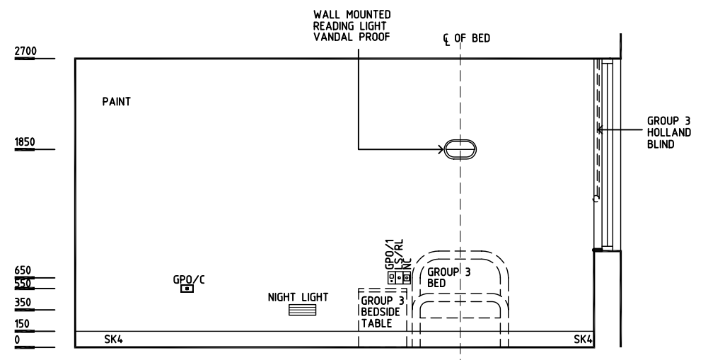
ELEVATION 4
