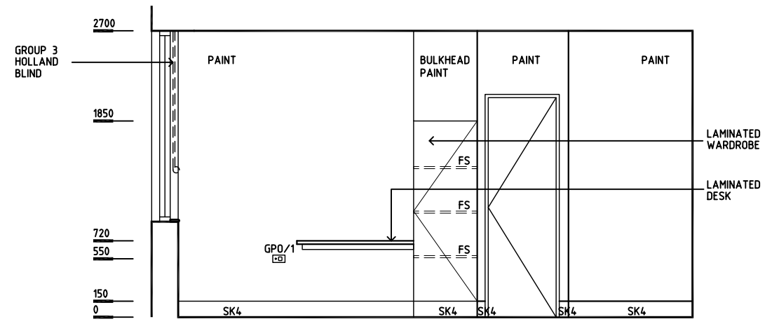
ELEVATION 2
