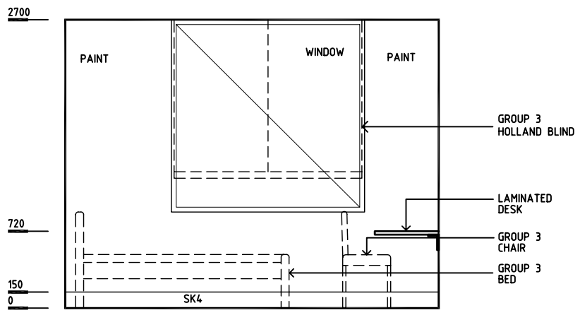
ELEVATION 1
