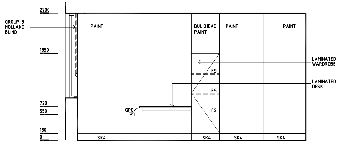
ELEVATION 2
