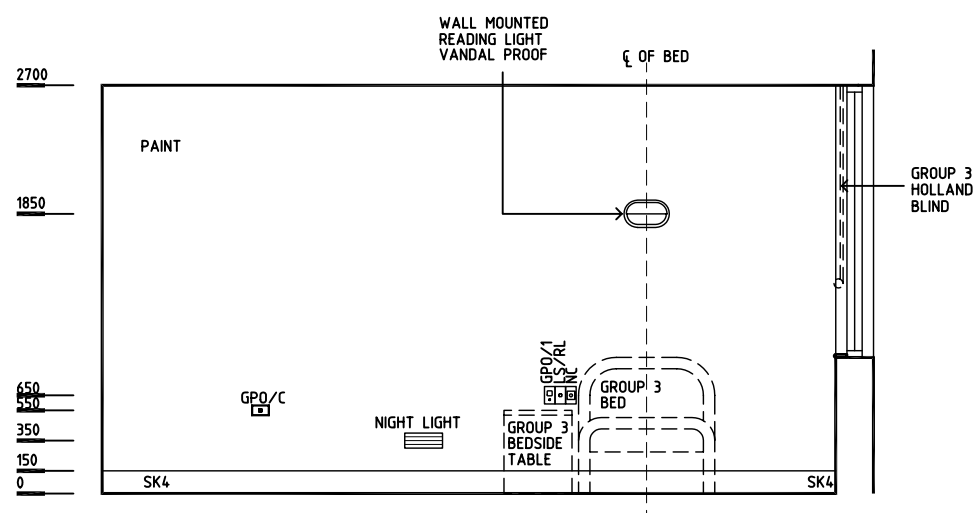
ELEVATION 4
