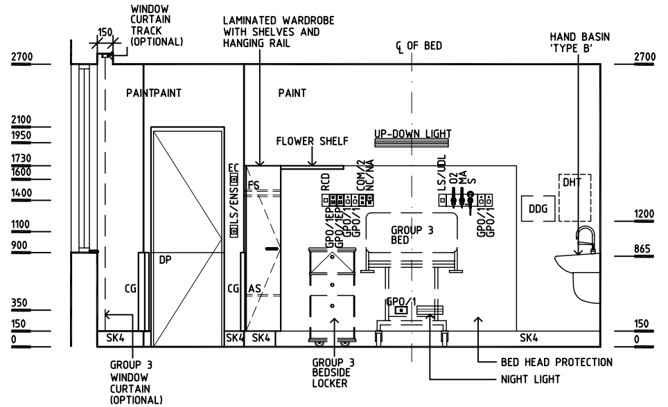
ELEVATION 2
