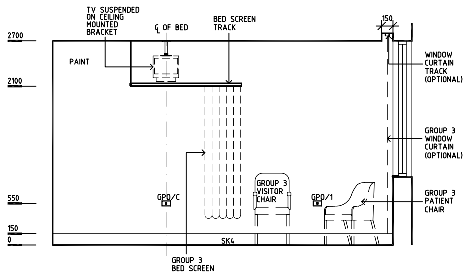
ELEVATION 4
