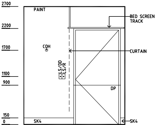
ELEVATION 1
