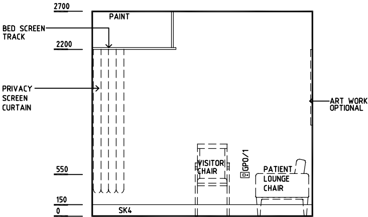
ELEVATION 2
