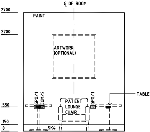
ELEVATION 3
