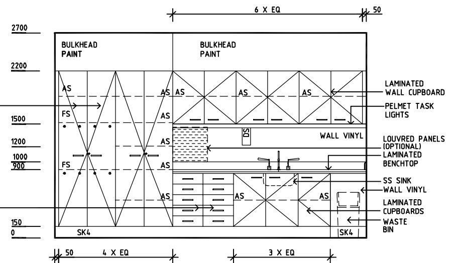
ELEVATION 2
