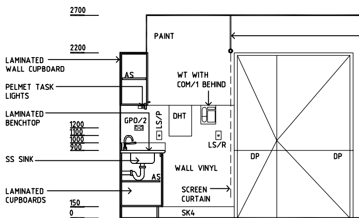
ELEVATION 3
