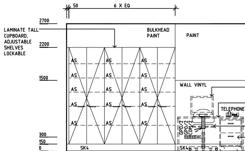
ELEVATION 1
