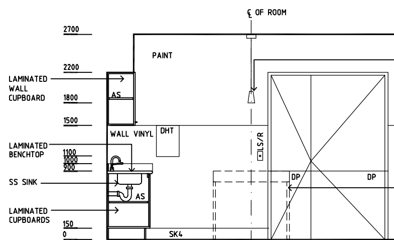
ELEVATION 3
