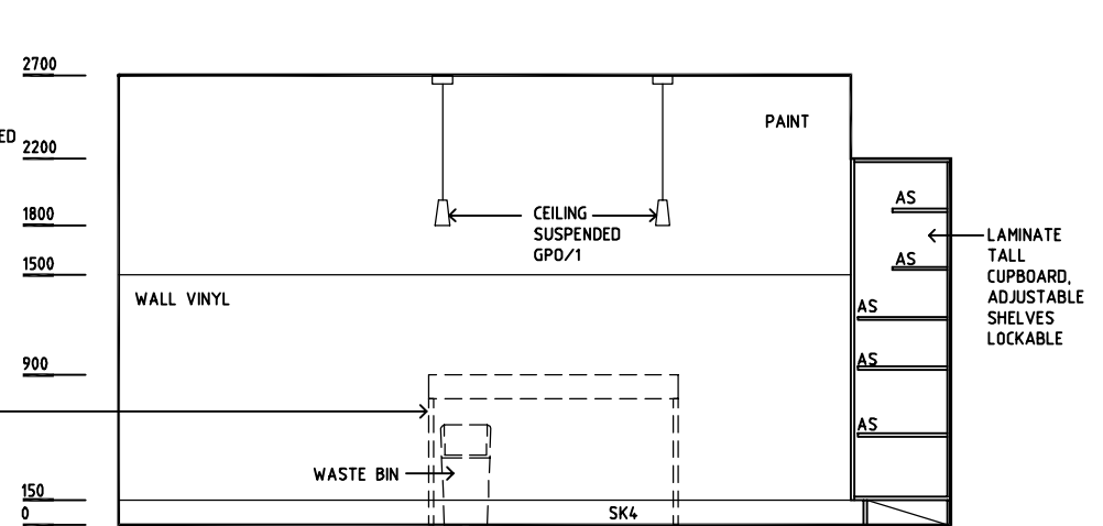
ELEVATION 4
