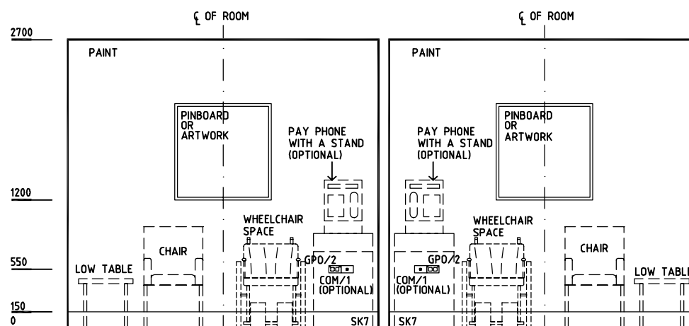
ELEVATION 4
