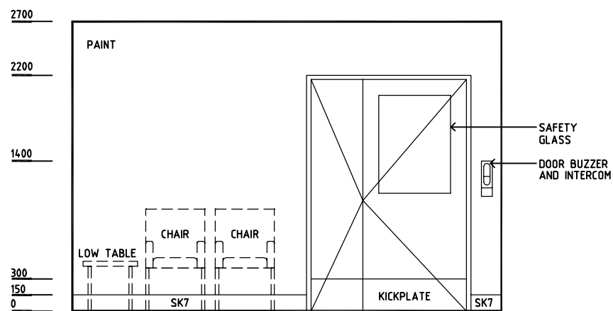
ELEVATION 1
