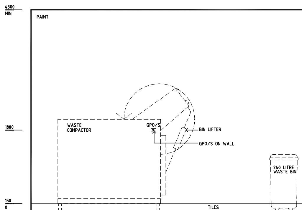
ELEVATION 1
