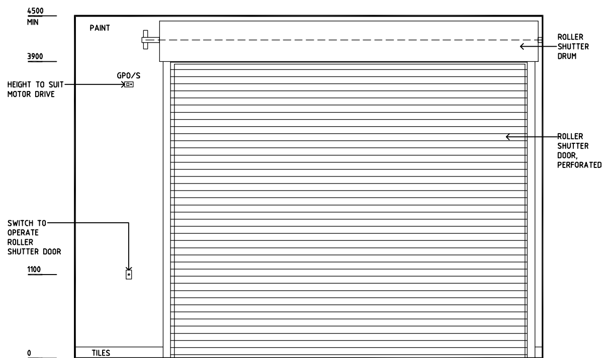
ELEVATION 3
