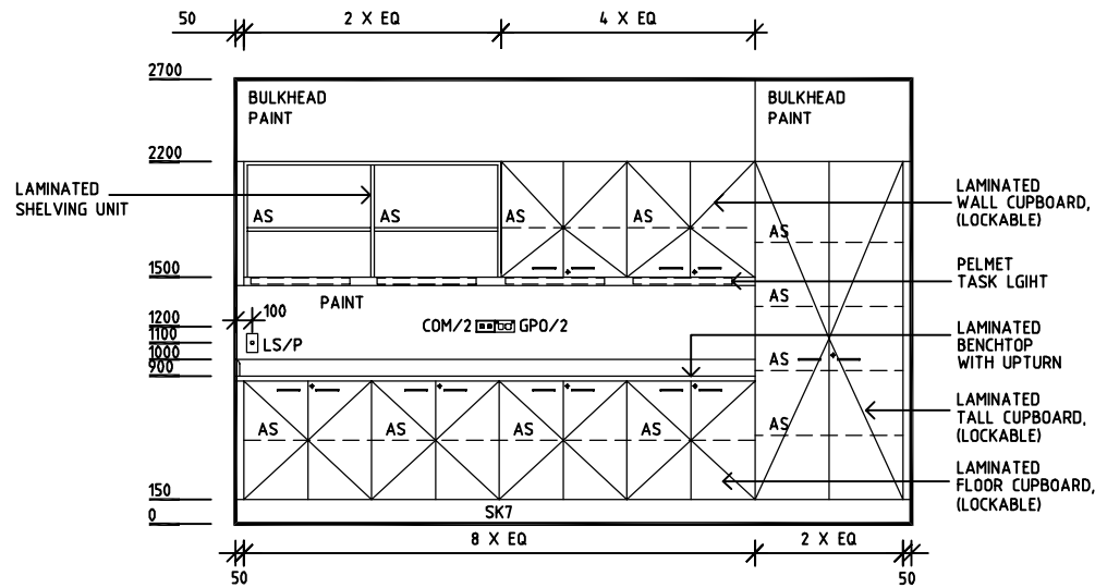
ELEVATION 2
