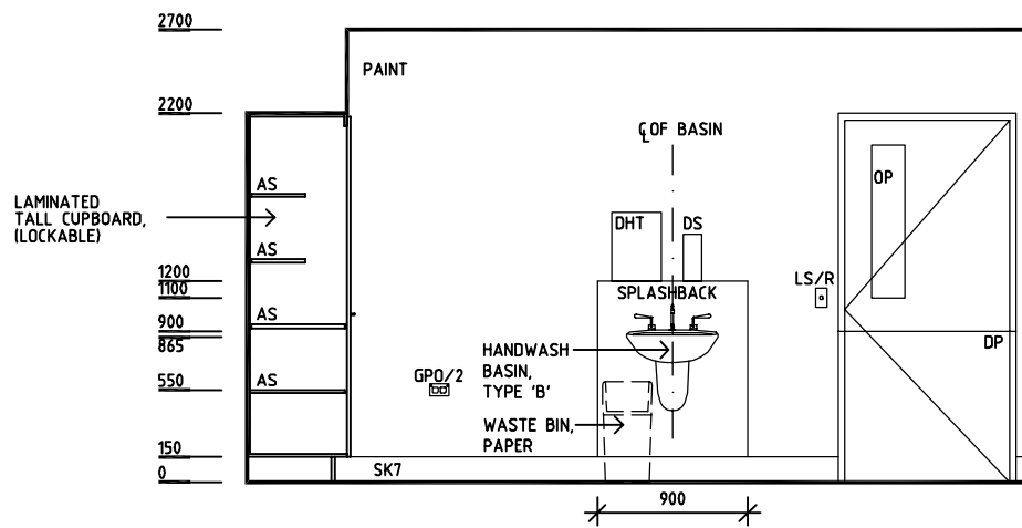
ELEVATION 3
