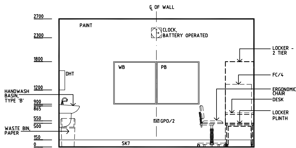
ELEVATION 4
