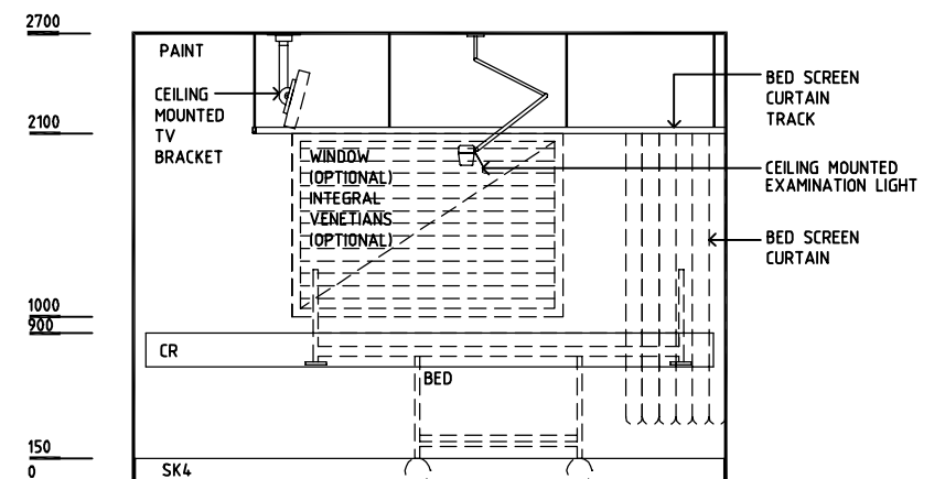
ELEVATION 4
