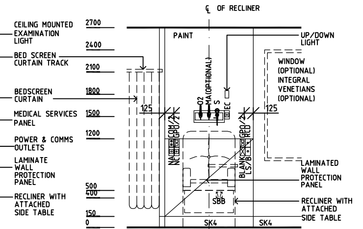
ELEVATION 5
