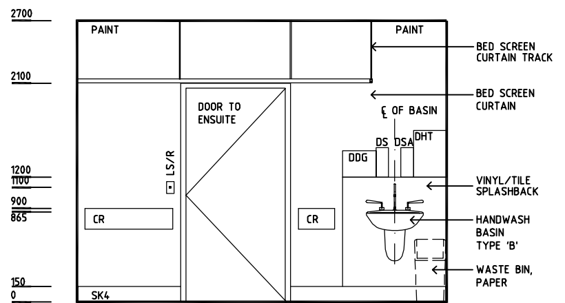
ELEVATION 2
