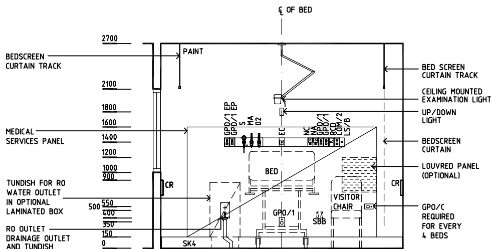
ELEVATION 1
