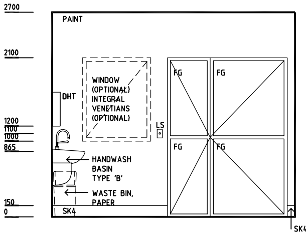
ELEVATION 3
