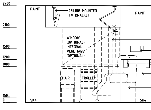
ELEVATION 4
