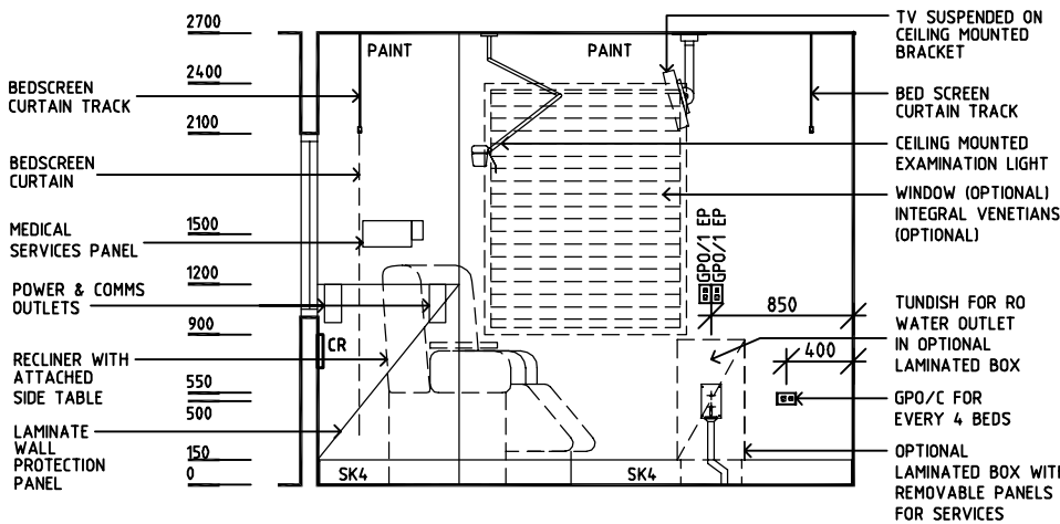
ELEVATION 1
