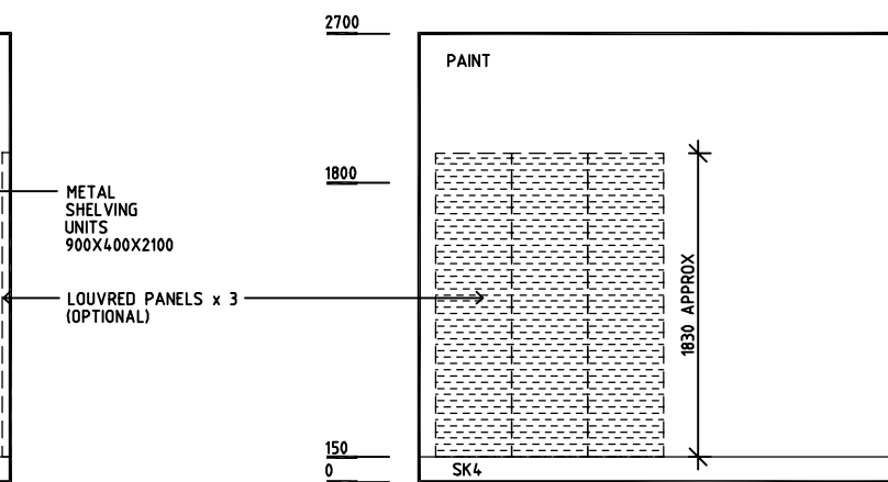
ELEVATION 2
