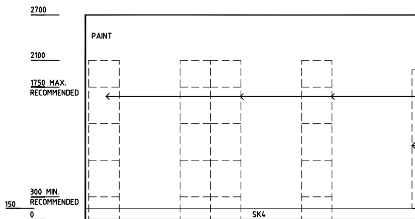
ELEVATION 1
