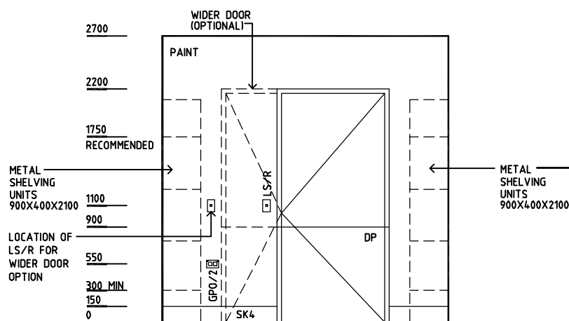
ELEVATION 3
