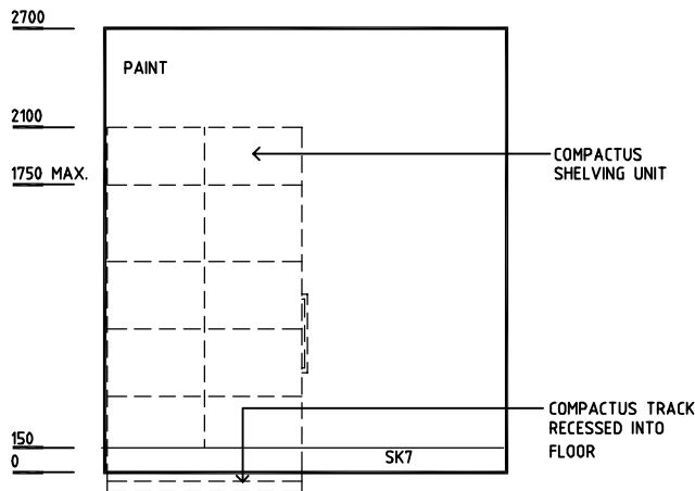
ELEVATION 2
