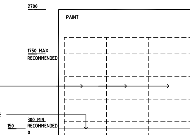
ELEVATION 4
