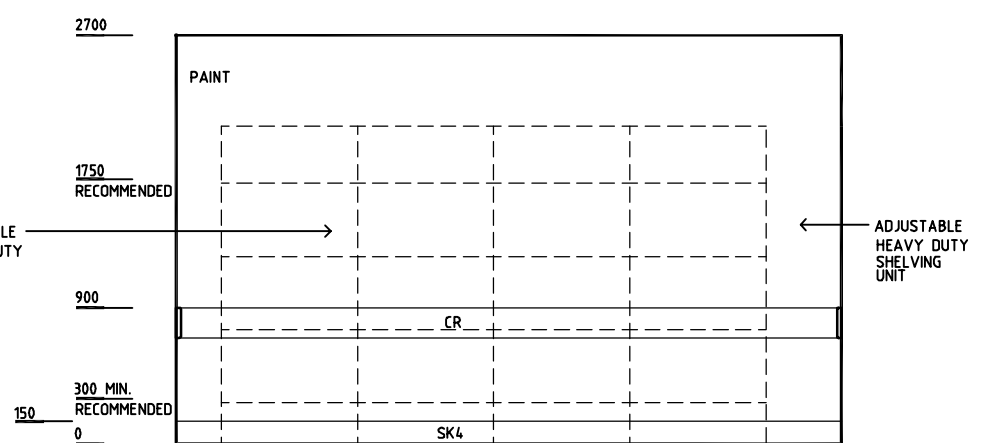
ELEVATION 4
