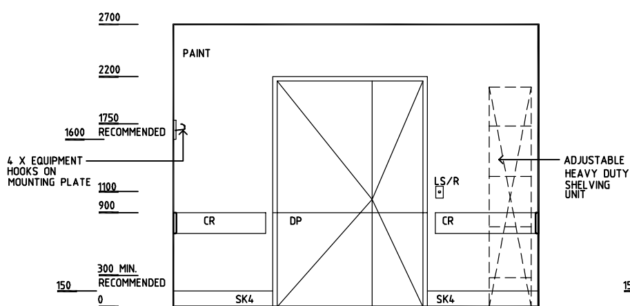
ELEVATION 3
