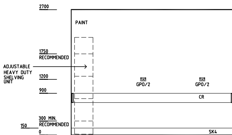
ELEVATION 1
