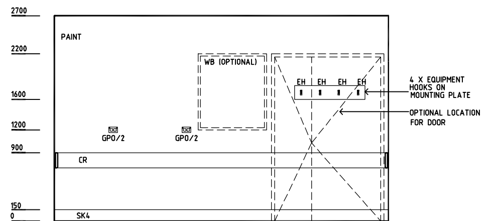
ELEVATION 2
