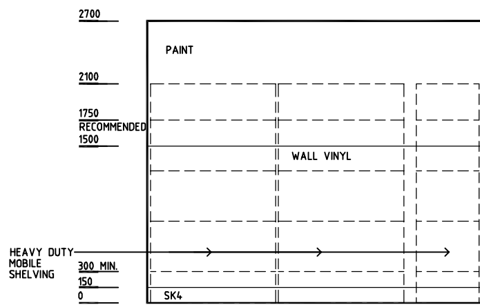
ELEVATION 1
