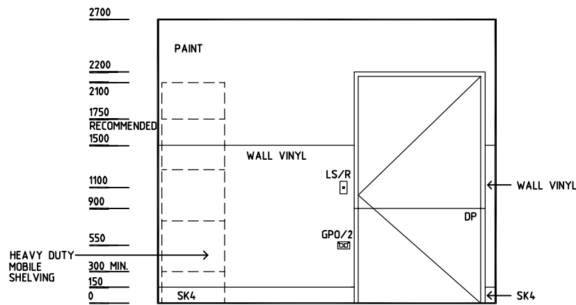
ELEVATION 3
