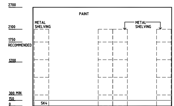
ELEVATION 4
