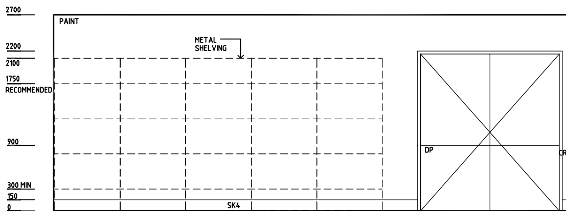
ELEVATION 1
