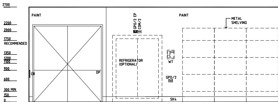
ELEVATION 3
