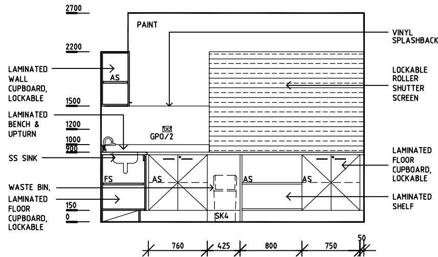
ELEVATION 2
