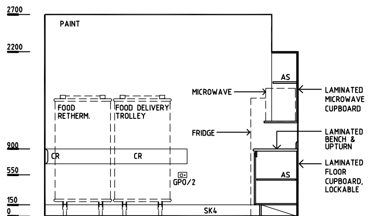
ELEVATION 4
