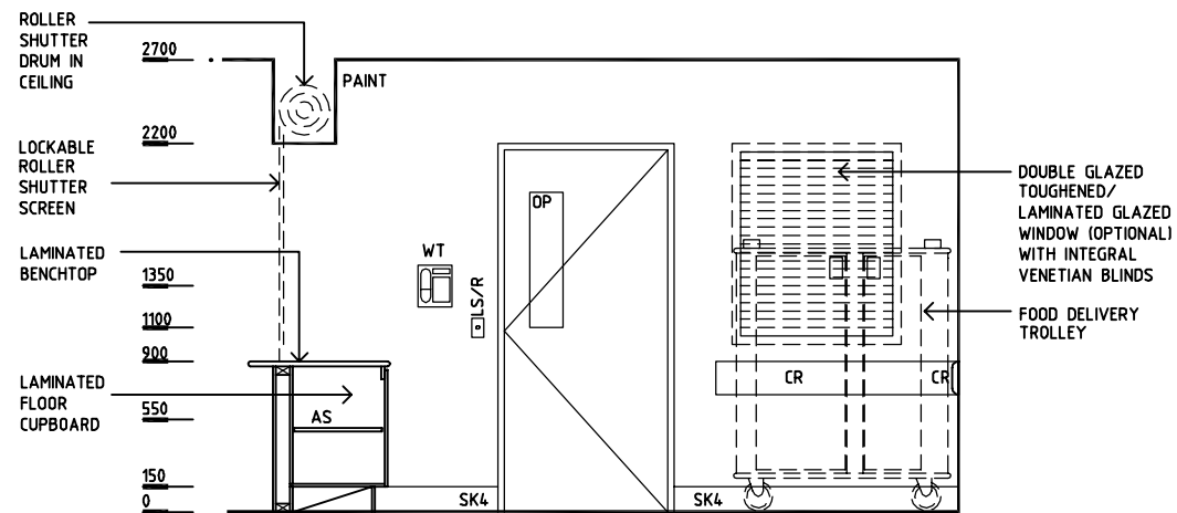
ELEVATION 3
