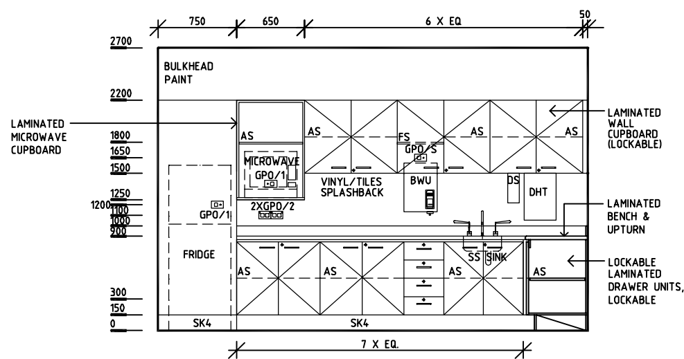
ELEVATION 1
